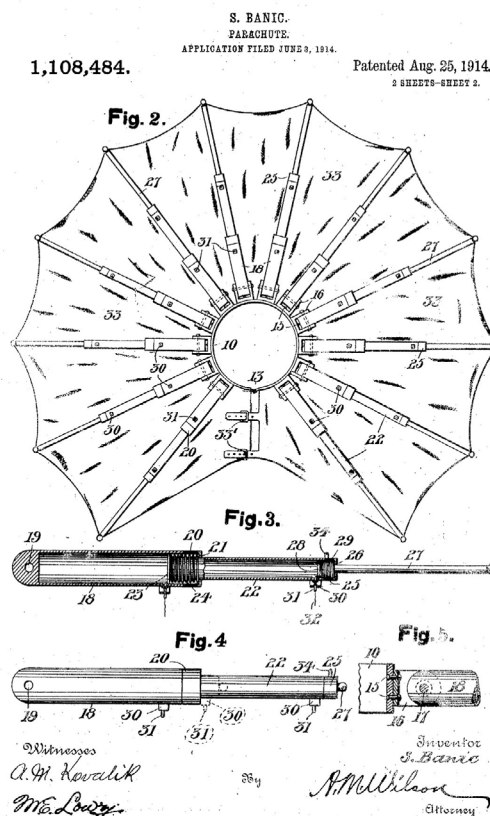
Nákres konštrukcie padáka, 1914
